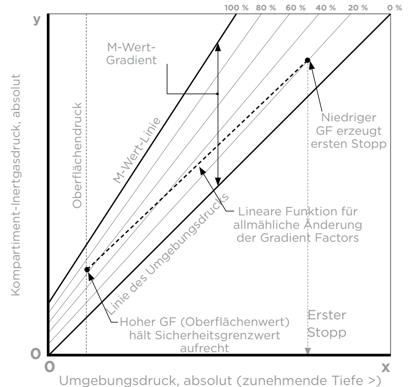
Druckdiagramm: Gradient Factors
